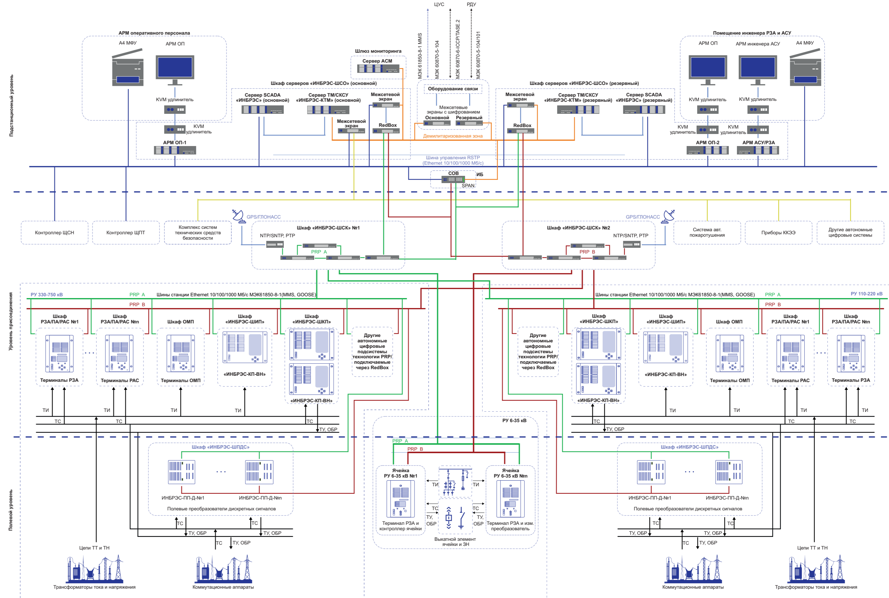
Рисунок 1 ПС 220-750 кВ
